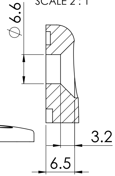
SECTION A-A SCALE 2 : 1
